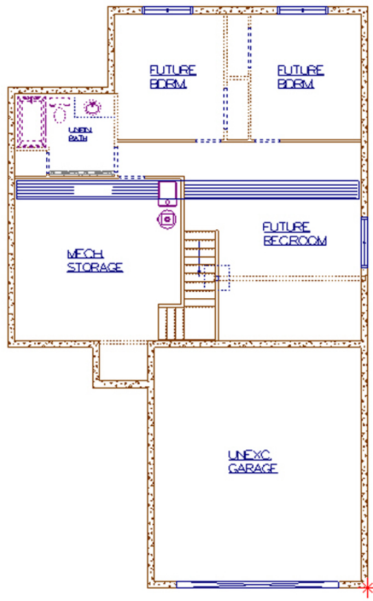
OPTIONAL BASEMENT PLAN
